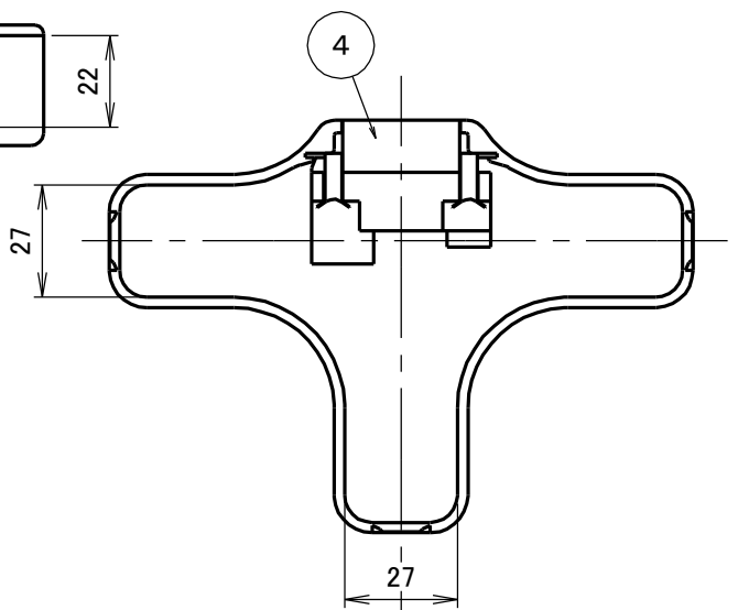
本体の内部寸法図 (1/2)
